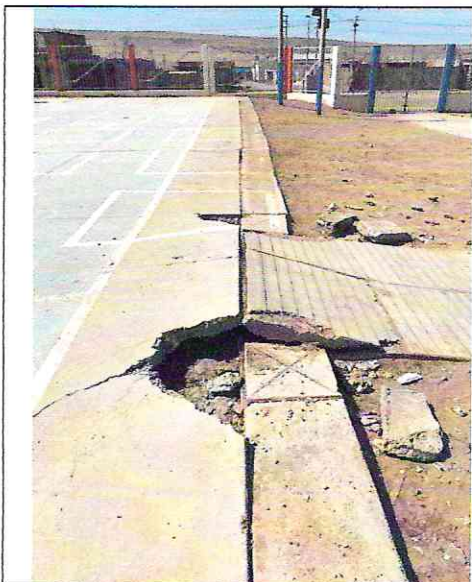
Imagen n° 21: Piso de losa deportiva con concreto colapsado.
