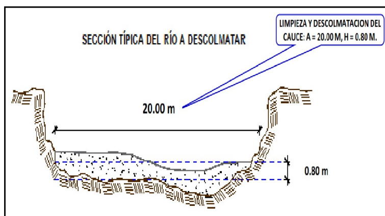
Imagen n.º 1 Sección Típica propuesta en la FTR
